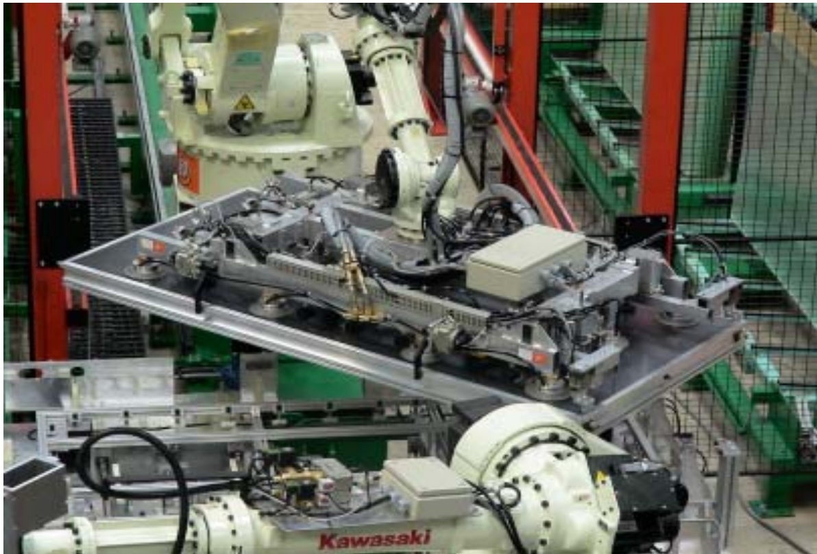
Abb. 19: Vollautomatisierte Fertigung von Sonnenkollektoren sorgt für ein hohes Qualitätsniveau und reduzierte Kosten. (Sun Master Energiesysteme GmbH, Kirchdorf).
