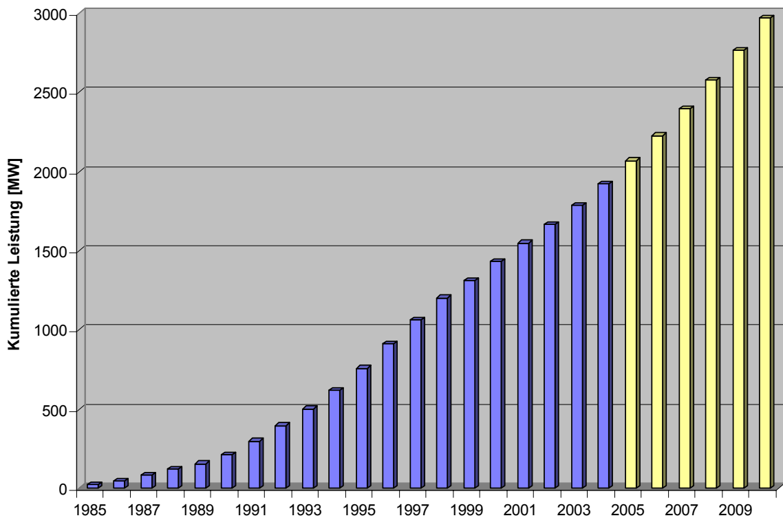
Abb. 28: Installierte Gesamtleistung im Jahr 2010 in Österreich 2,9 GW. Gesamtwärmeertrag der Anlagen: 1.453 GWh. Moderates Szenario.
