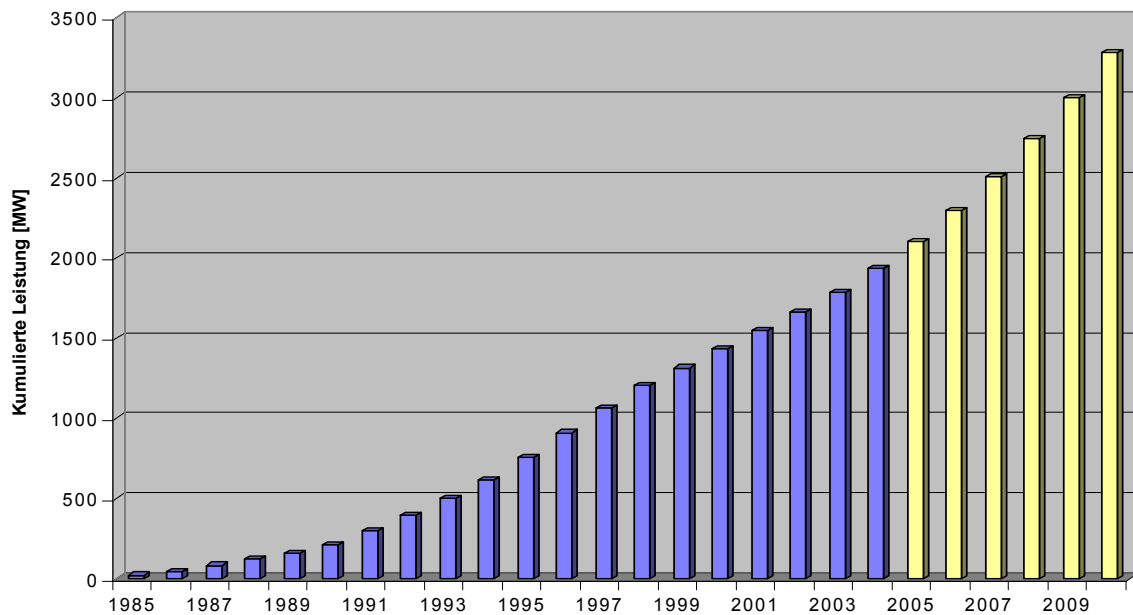
Abb. 31: Installierte Gesamtleistung im Jahr 2010 in Österreich 3,2 GW. Gesamtwärmeertrag der Anlagen: 1.586 GWh. Ambitioniertes Szenario.
