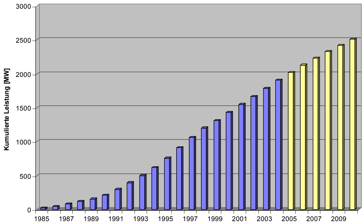
Abb. 25: Installierte Gesamtleistung im Jahr 2010 in Österreich 2,5 GW. Gesamtwärmeertrag der Anlagen: 1.229 GWh. BAU -Szenario
