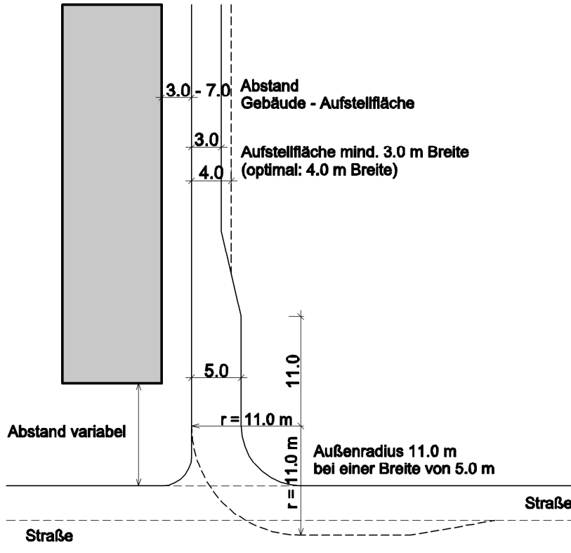
Abbildung 4-1: Darstellung Platzbedarf und Kurvenradius für Anlieferung
