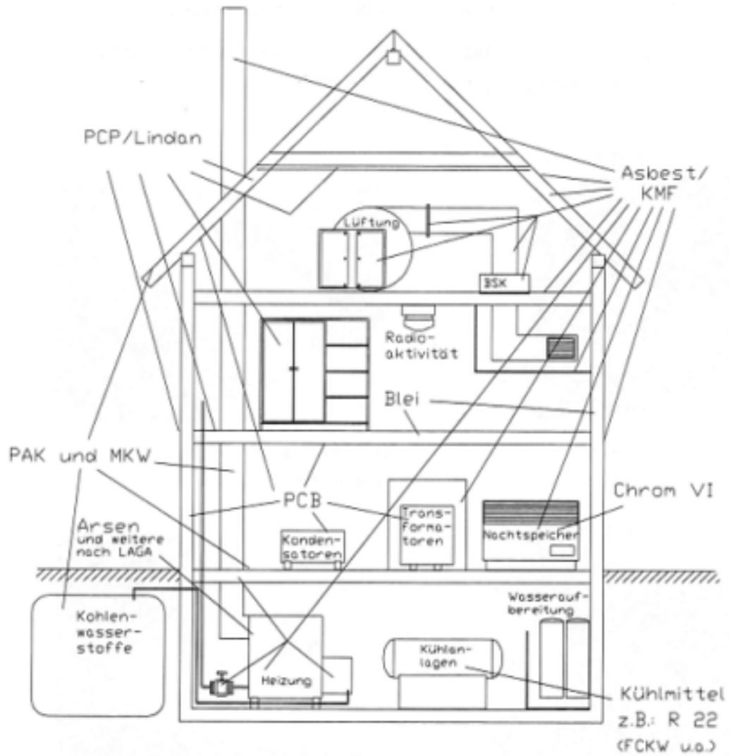
Abbildung 2-1: Übersicht möglicher Fundstellen schadstoffhaltiger Produkte (Quelle: Kratochwil A., et al: "Schadstoffe bei Abbruchplanungen – Gefährdungseinschätzung, Abbruchplanung und Umsetzung", VDI Jahrbuch 2000-2001 [12])
