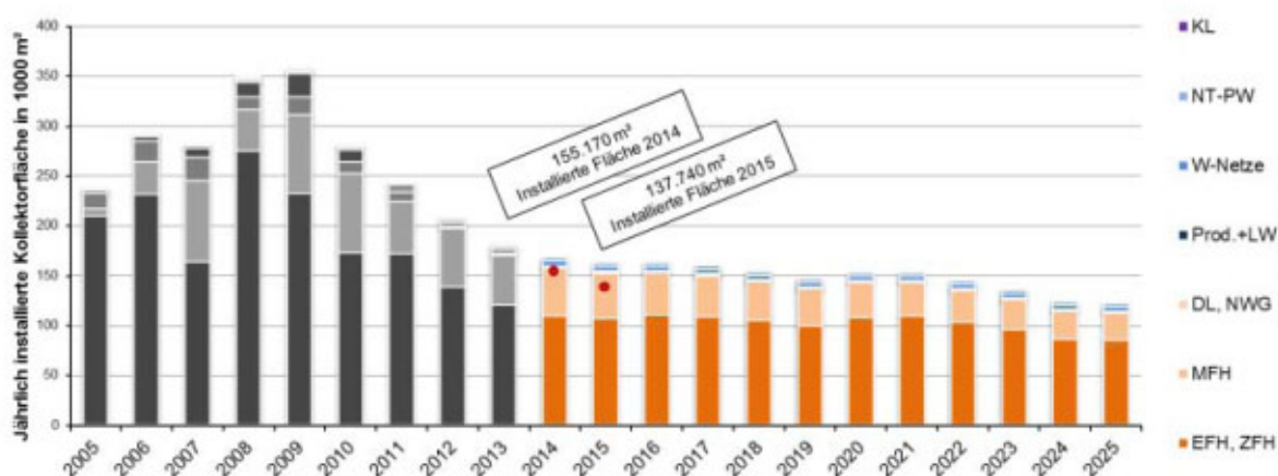
Abbildung 8.13: Kollektorflächenentwicklung (Flach- und Vakuumröhrenkollektoren) und Verteilung nach Anwendungssektoren im Szenario „Business as Usual“. Grau dargestellt sind hier die bereits in der Vergangenheit jährlich umgesetzten Kollektorflächen, färbig dargestellt sind die Roadmap Prognosen bis 2025. Für die Jahre 2014 und 2015 ist jeweils die tatsächlich installierte Kollektorfläche eingetragen.
