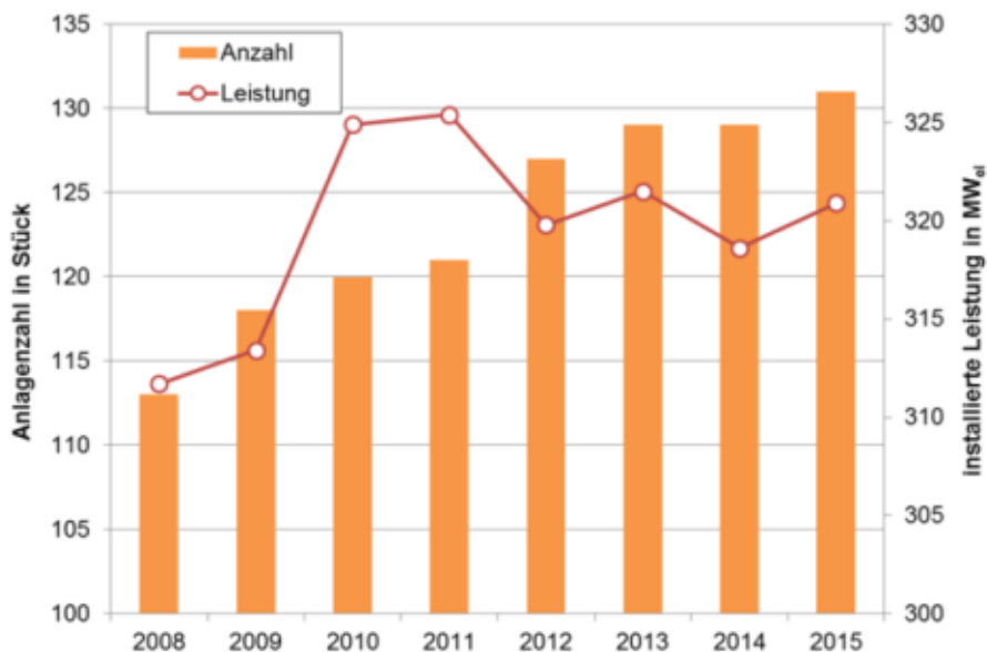
Abbildung 6.7: Bestandentwicklung aktiver Ökostromanlagen mit Brennstoff fester Biomasse und installierter Leistung in MW el . Datenquelle: OeMAG (2016)
