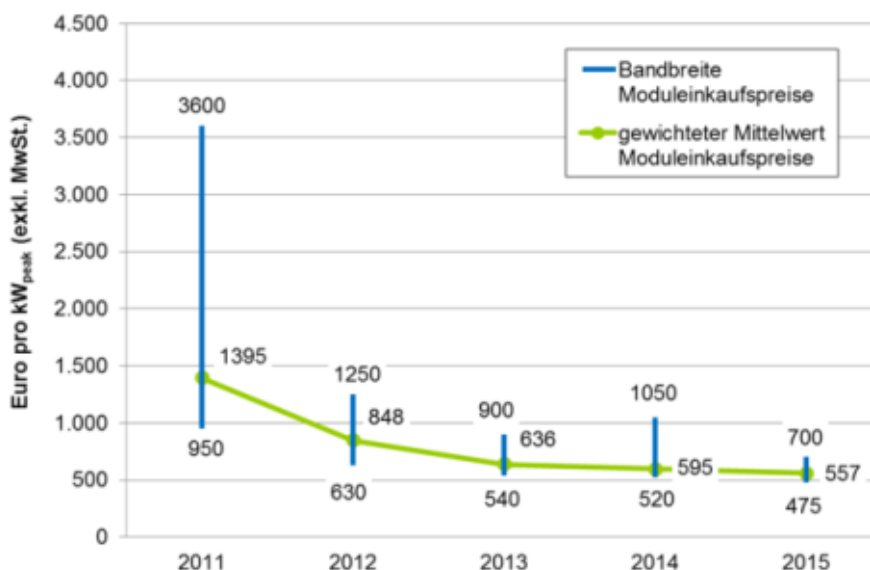
Abbildung 7.7: Mittelwert und Bandbreite der Moduleinkaufspreise von Anlagenerrichtern und Planern der Jahre 2011 bis 2014, Werte exkl. MwSt.; Anzahl der Nennungen: 2011: n=26, 2012: n=28, 2013: n=32, 2014: n=28; Quelle: Erhebung Technikum Wien.
