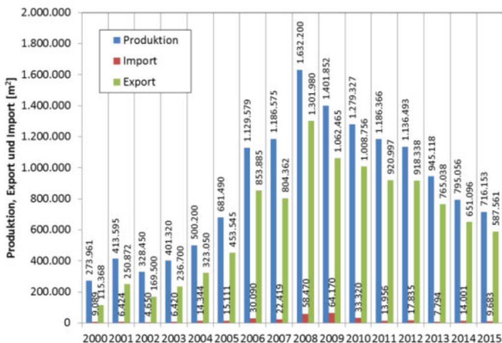
Abbildung 8.3: Produktion, Export und Import von thermischen Kollektoren in Österreich in den Jahren 2000 bis 2015. Quellen: bis 2006: Faninger (2007), ab 2007: AEE INTEC
