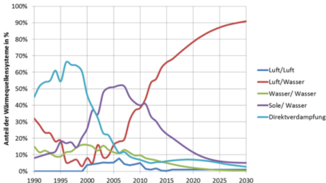
Abbildung 9.12: Trendszenario für die Marktanteile der Wärmequellsysteme von Heizungswärmepumpen und Wohnraumlüftungswärmepumpen. Bis 2015: empirisch erhobene Marktentwicklung; ab 2016: Szenarienwerte. Quellen: bis 2006: Faninger (2007), von 2007 bis 2015: Biermayr et al. (2016)
